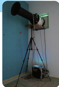
醍醐寺の家 気密測定
