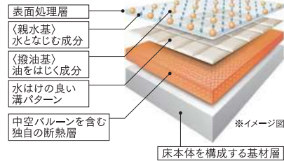
キレイサーモフロア断面図
